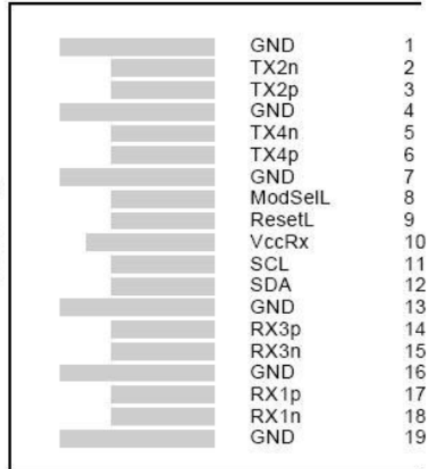
Bottom Side
