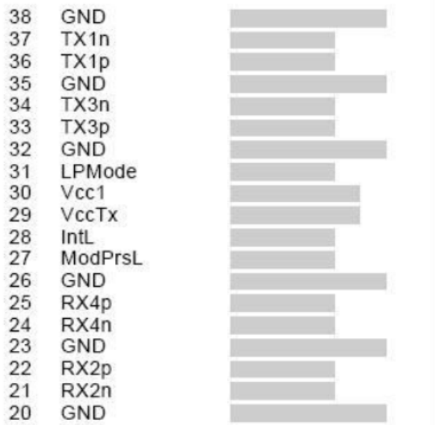
Top Side
